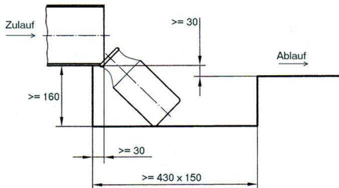
Bild 1 – Mindestmaße der Probenahmereinrichtung
