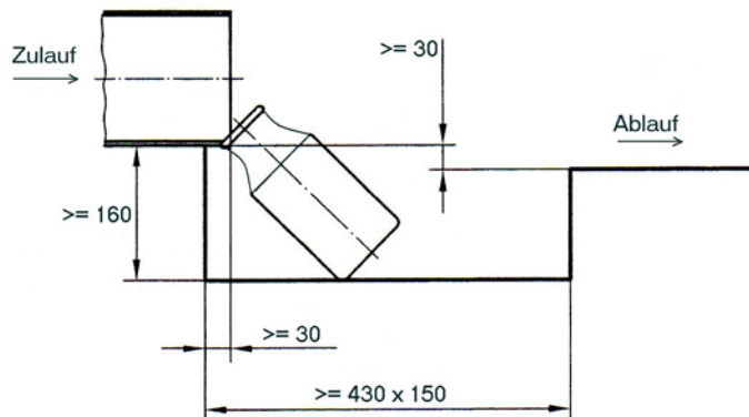
Bild 1 – Mindestmaße der Probenahmeeinrichtung
